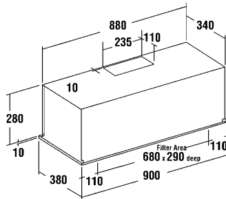
ECH-900-1-T/B
