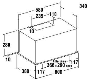
ECH-800-2-T/B
