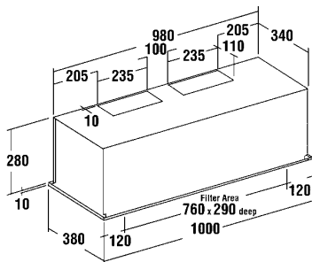
ECH-1000-2-T/B
