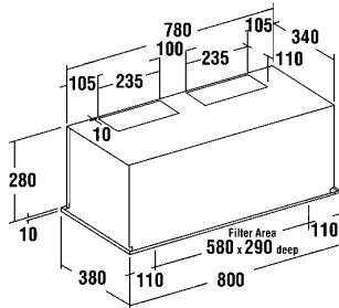
ECH-1000-2-T/B
